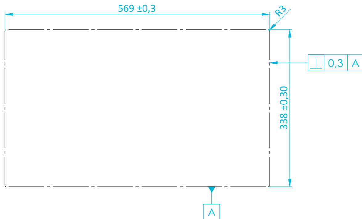
Einbau-Ausschnitt OPC8024 Mounting-Cutout OPC8024
